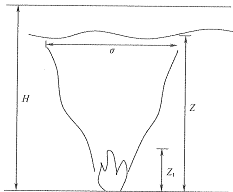
图 10 轴对称型烟羽流
