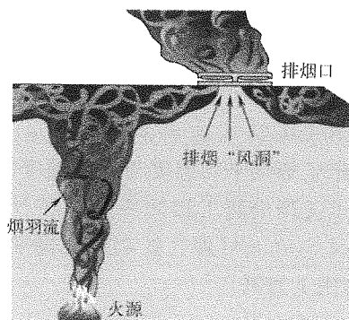
图 15 排烟口的最高临界排烟量示意图
