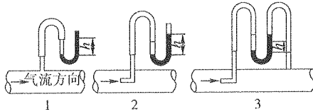
图 19 用 U 形管压力计测定风压
