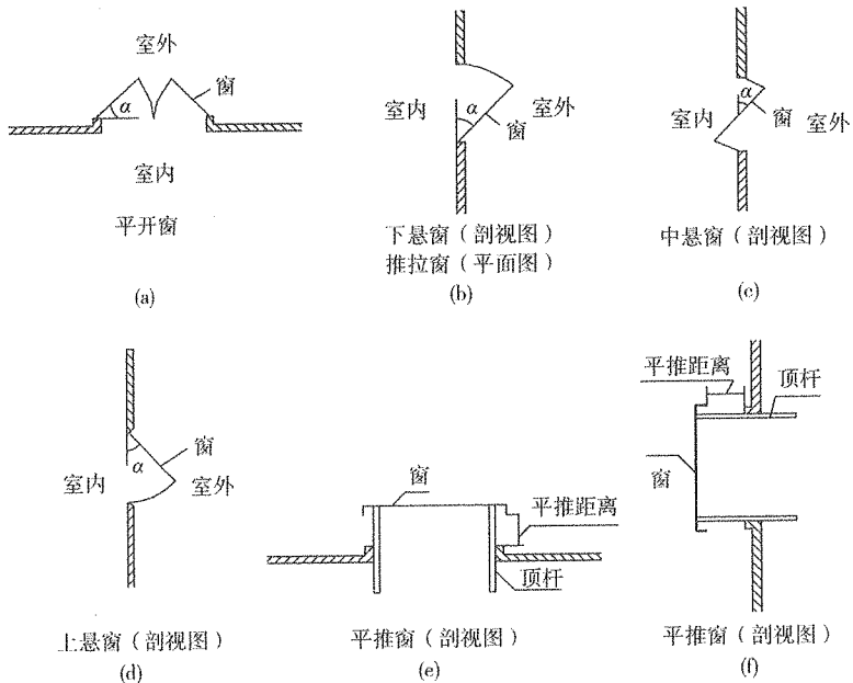
图 6 可开启外窗的示意图
