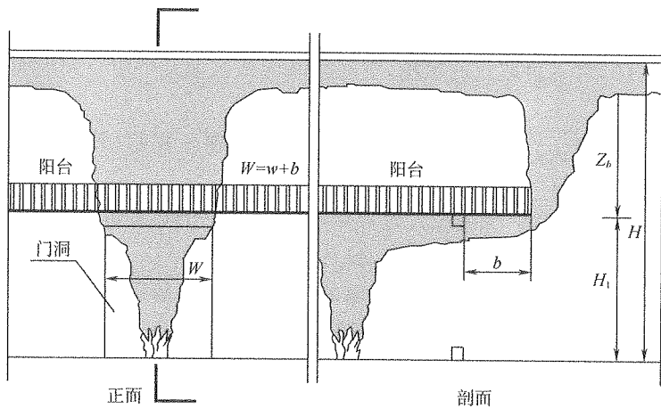
图 11 阳台溢出型烟羽流
